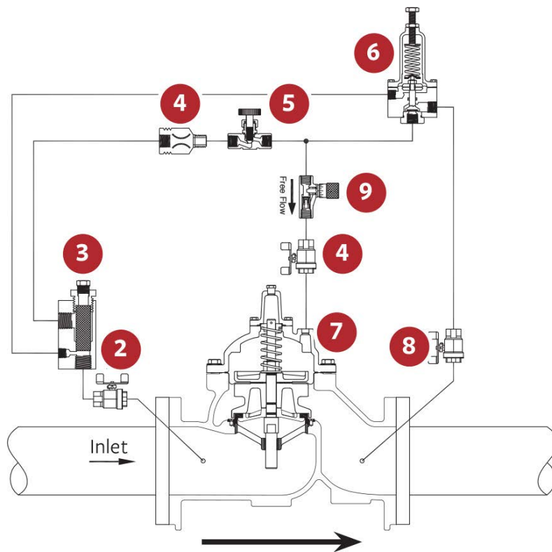
Schematic A-0423F
