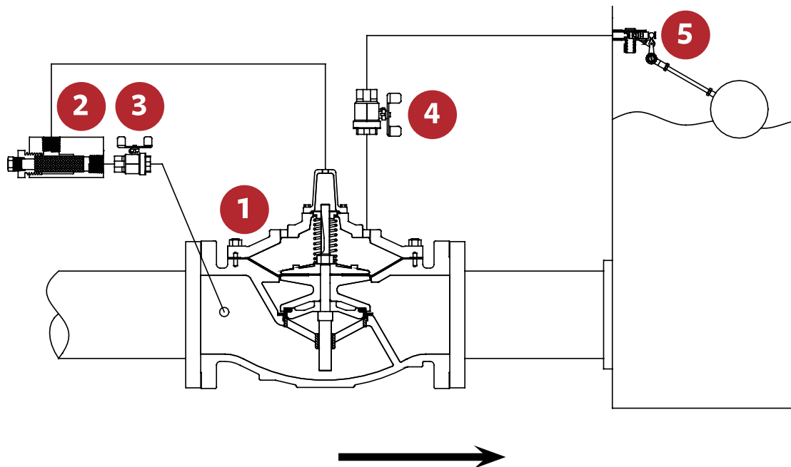
FIG. 2 Schematic A-0593C
