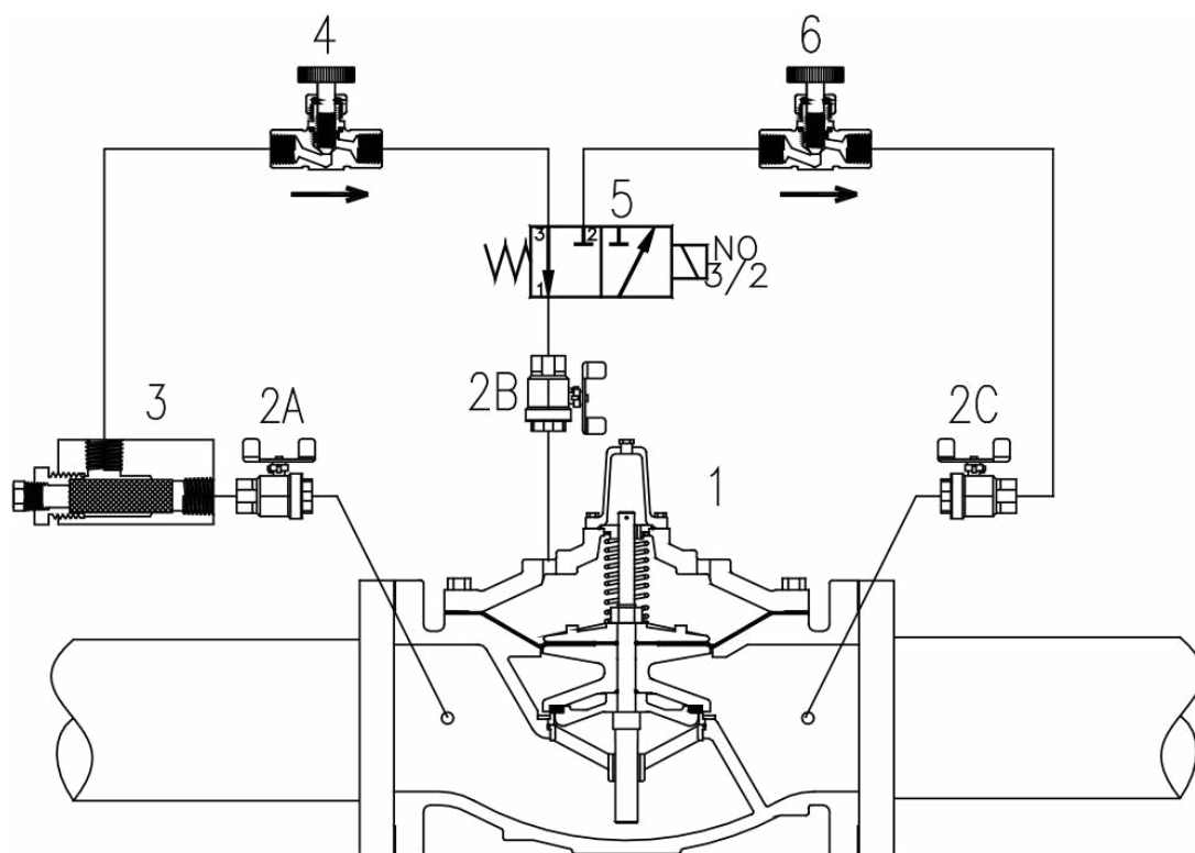
FIG. 2 Schematic A-0593C
